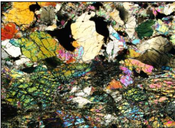
Figure 14 - Cristaux de la lherzolite diversement fracturés aux débris peu déplacés (E. de Lherz)
