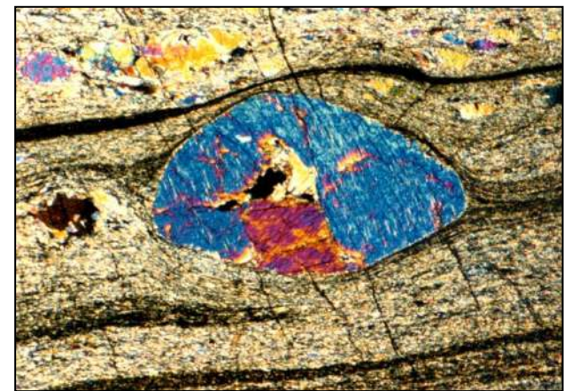
Figure 15 - Cristaux de la lherzolite finement broyés et déplacés (Turon de la Técoùère, Pyr.-Atl.)
