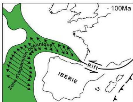
Figure 25 – Les deux dernières étapes de l'ascension des lherzolites en carte (d'après M. Mattauer, 1989). De -107 à -85 Ma : dans les tréfonds du rift (sillon des flyschs nord-pyrénéens) lors de la « dérive » de l'Ibérie par rapport à l'Europe. De 85 à 40 Ma : dans la zone nord-pyrénéenne lors du rapprochement de l'Ibérie et de la surrection de la chaîne pyrénéo-provençale.
