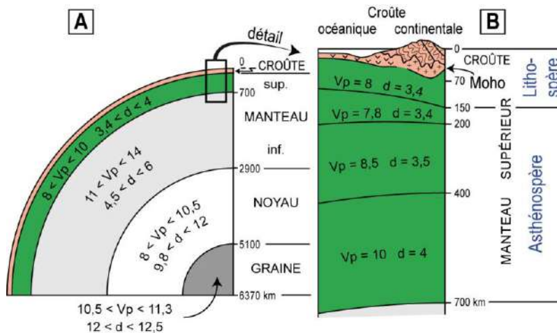
Figure 16 – Place du manteau supérieur, en vert, dans le globe terrestre (A) et détail de l'organisation du manteau supérieur (B). d : densité moyenne des roches ; Vp : vitesse de propagation des ondes sismiques P en km/s (d'après Foucault & Raoult, Dictionnaire de Géologie, Dunod, 2003).
