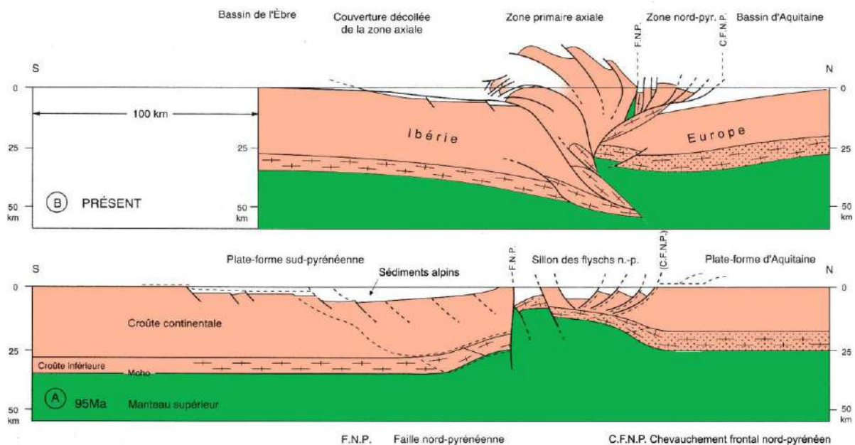
Figure 18 – Les deux dernières étapes de l'ascension du manteau supérieur lherzolitique en coupe (d'après Roure & al., 1989, Tectonics , 8, 1, 41-50).
