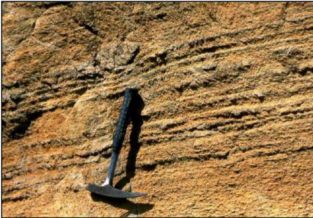
Figure 6 - Lits de webstérite plissés dans la lherzolite (Etang de Lherz).
