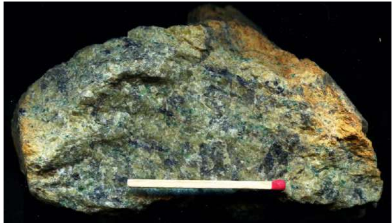
Figure 4 - Echantillon de lherzolite fraîche et sa croûte d'altération (Lherz).
