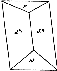
Fig. 11. Sphène de granites.
