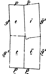
Fig. 6. Projection sur un plan perpendiculaire à l'axe a d'une extrémité d'une macle de l'Esterel. L'angle rentrant de la fig. 4 a disparu.
