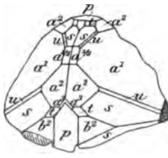
Fig. 64. Pyrite d'Arnave.
