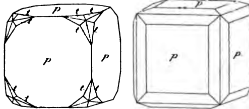
Fig. 8 et 9. Fluorine de Romanèche.
