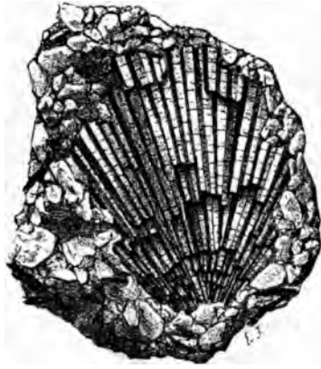
Fig. 9. Béryl de Pont-Percé. (Réduction de 1/2.)
