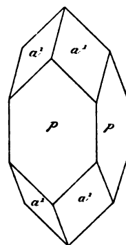
Fig. 7. Pyrite de Barbin.
