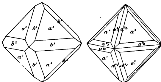
Fig. 11 et 12. Galène de Pontgibaud.
