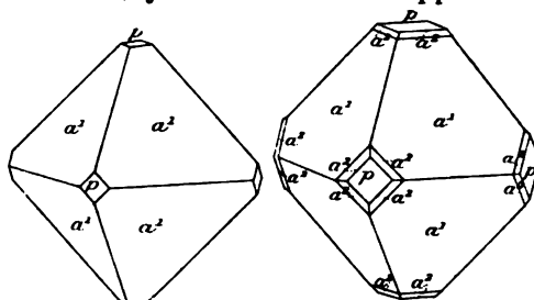
Fig. 49 et 50. Pyrite de Betchat.
