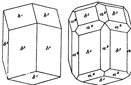
Fig. 13 et 14. Panabase allongée suivant un axe ternaire, (Framont.)
