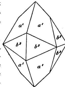
Fig. 47. Pyrite de Saint-Béat.
