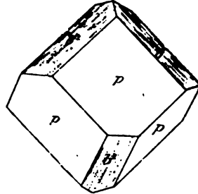
Fig. 11. Chabasia de Cambo.
