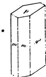
Fig. 1. Dyscrasite de Sainte-Marie-aux-Mines.
