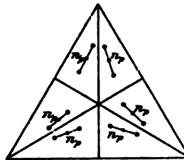
Fig. 3. Section a^1 (0001) du type II.
