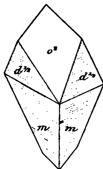
Fig. 6. Sphène (spinthère de Maronne). (Type IV.)
