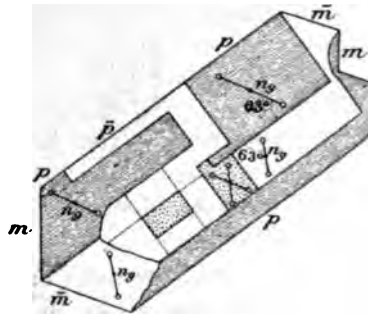
Fig. 3. Face g^1 (010) de l'harmotome à disposition enchevêtrée (Vialas).
