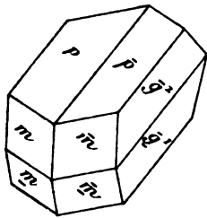
Fig. 5. Andésine de Boulouris (macle de l'Esterel).
