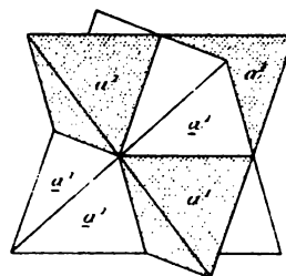
Fig. 11. Panabase. Macle par entre-croisement.
