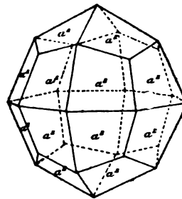
Fig. 2. Trapézoèdre de leucite.
