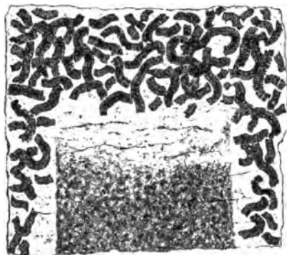
Fig. 49. Lame mince d' adulaire chloritée du Dôme du Goûter, montrant des groupements vermiculaires de ripidolite ( helminthé ) localisés sur les bords du cristal, qui au centre ne renferme que des lamelles enchevêtrées du même minéral. (Grossissement de 20 diamètres. Lumière naturelle.)
