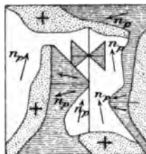
Fig. 11. Section de la macle de Marburg perpendiculaire à l'axe a (Si-miouse).
