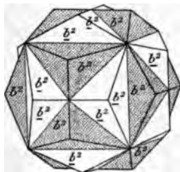
Fig. 43. Maclé de Lurdé.
