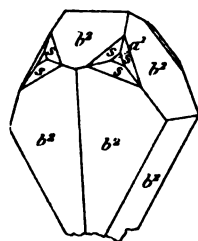
Fig. 16. Pyrite d'Allevard.
