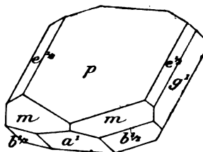
Fig. 46. Orthose sodique des enclaves du Capucin.
