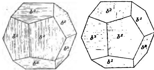
Fig. 4 et 5. Stries sur les deux types de dodécèdres pentagonaux de pyrite.
