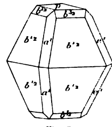
Fig. 7. Soufre de Saint-Boès.
