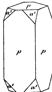
Fig. 19. Pyrite d'Itsatsou.
