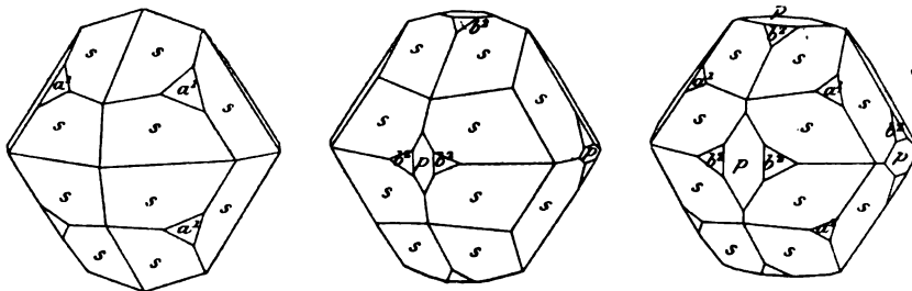
Fig. 60 à 62. Pyrite de Betchat.
