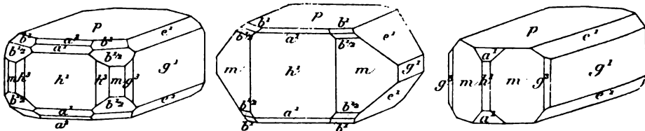
Fig. 1 à 3. Bourbonite.
