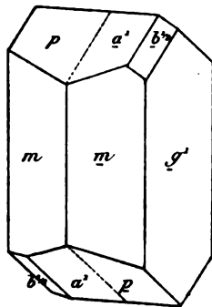
Fig. 9. Macle de Carlsbad par accolement (orthose).
