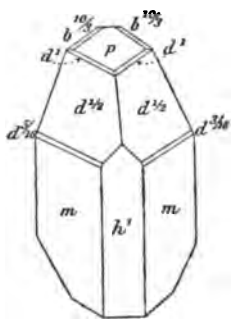
Fig. 16. Sphène du lac Lovit.
