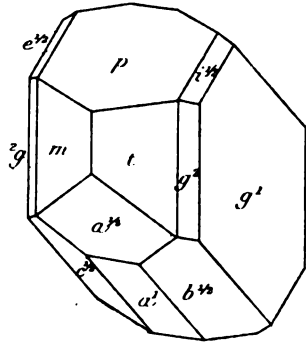
Fig. 9. Albite de l'Oisans (Type II).
