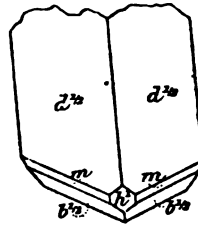
Fig. 22. Sphène des cendres du Croustet.
