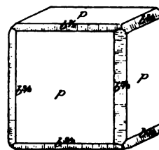
Fig. 8. Pyrite de Huelgoat.
