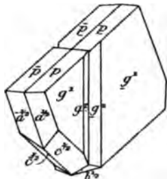
Fig. 20. Macle du Roc Tourné, clivée suivant les faces p .
