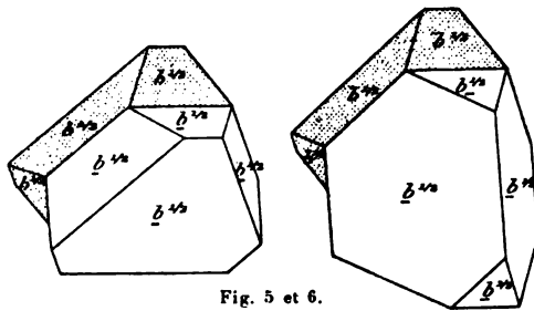
Fig. 5 et 6. Chalcopryrite. Macle suivant b^{1/2} (111) .
