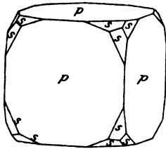
Fig. 58. Pyrite de Betchat.
