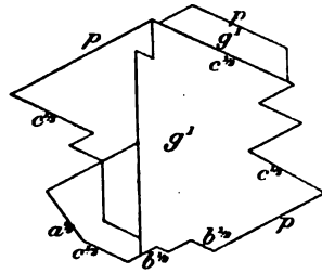
Fig. 32. Empilement suivant l'axe vertical de cristaux d'albite présentant la triple macle. Silhouette g^1 (010).
