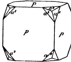
Fig. 2. Analcime de la Réunion.
