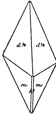
Fig. 17. Sphène de la syénite néphélinique de Pouzac.
