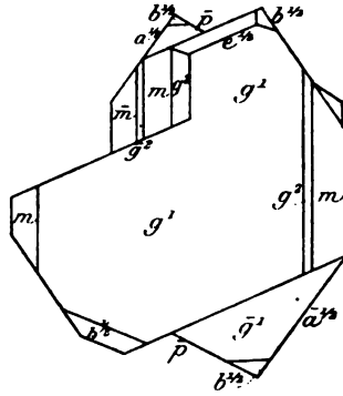
Fig. 24. Groupement d'orthose (Four-la-Brouque)
