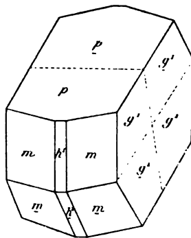
Fig. 5. Morvenite de la mine d'Anglas.
