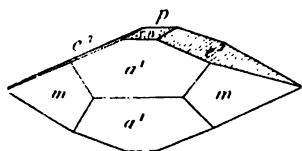
Fig. 7. Mispickel de Saint-Prix.
