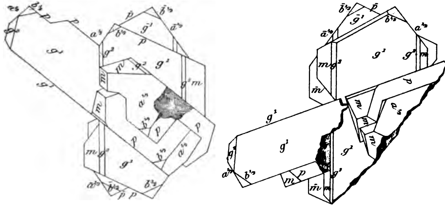
Fig. 22 et 23. Groupement d'orthose. La fig. 23 représente le même groupement que la fig. 22, après rotation de 90^\circ autour de l'arête pg^1 de la macle de Baveno.
