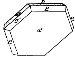
Fig. 27. Maclé suivant \alpha^4 de la galène de Bielsa.
