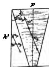
Fig. 3. Face g^1(010) de la brewsterite de Baréges.
