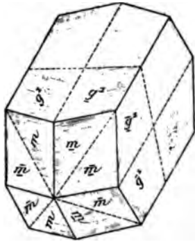
Fig. 14. Macle de Marburg sans angles rentrants (Saint-Jean-le-Centenier).
