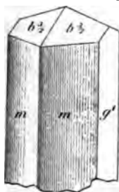
Fig. 7. Stibine de Saint-Mary- le-Plain.
