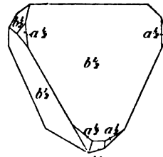
Fig. 4. Chalcopryrite. Forme commune.
