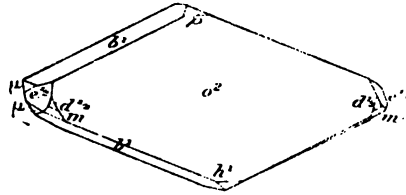
Fig. 10. Sphène du lac Noir (Type VII).
