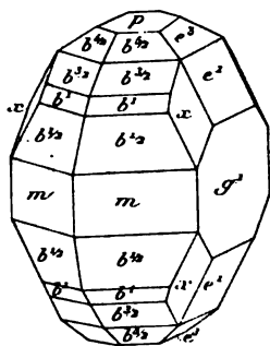
Fig. 8. Soufre de la Cendrière de Trépail.
