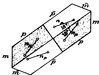
Fig. 12. Section g^1 (face extérieure) de la macle de Marburg.
