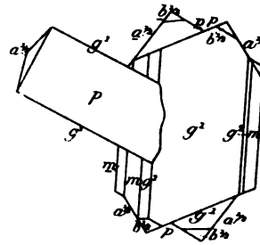
Fig. 25. Groupement d'une macle de Carlsbad et d'un cristal simple.
