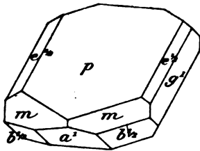
Fig. 8. Type VI. Orthose aplatis suivant p (001).
