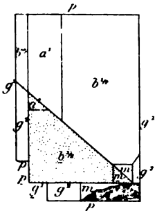
Fig. 9. Projection, sur un plan perpendiculaire à l'axe a , du groupement d'une maclé de Baveno et d'un cristal simple (Batz).
