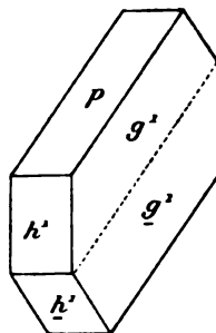
Fig. 16. Macle de la morvenite du mont Simieuse.
