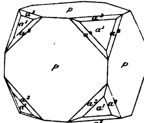
Fig. 59. Pyrite de Betchat.
