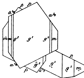
Fig. 26. Groupement d'une macle de Carlsbad et d'une macle de Baveno.
