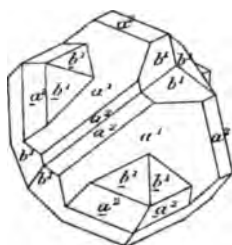
Fig. 10. Panabase. Macle suivant a^1 .
