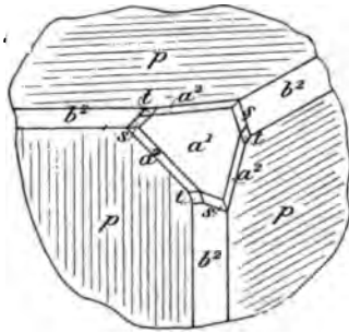
Fig. 63. Pyrite d'Arnave.
