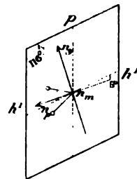
Fig. 2. Orthose déformée.
