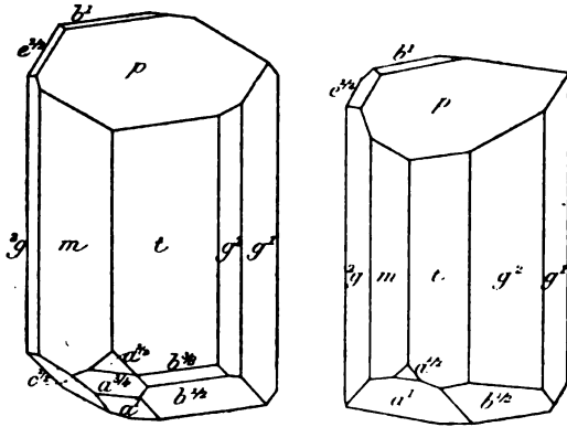
Fig. 3 et 4. Albite de l'Oisans (Type I).
