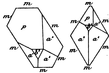
Fig. 7. Fig. 8. Projection, sur la base, de deux cristaux de béryl à sommets dissymétriques (La Villelder).
