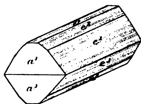
Fig. 3. Mispickel de la Villelder.
