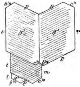
Fig. 3. Macle de Carlsbad avec accolement suivant une face de la zone verticale perpendiculaire à g^1 . (Silhouette de g^1 .)
