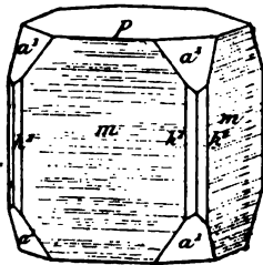
Fig. 4. Apophyllite de Bou Serdou.
