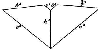
Fig. 9. Section g^2 (010) de la maclé suivant h^1 (100) d'un cristal du type VI. (Lac Noir.)
