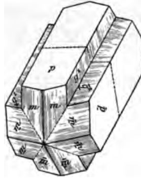
Fig. 3. Macle de Périer.
