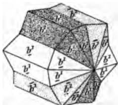
Fig. 3. Salmiac de la Ricamarie. Macle de trois individus.
