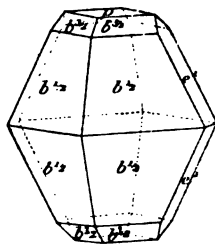
Fig. 6. Soufre de Saint-Boès.
