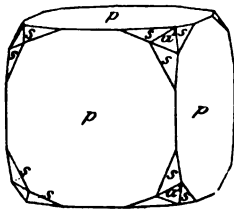
Fig. 21. Pyrite.
