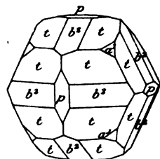
Fig. 9. Pyrite de Huelgoat.
