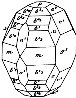
Fig. 9. Soufre des Malines.
