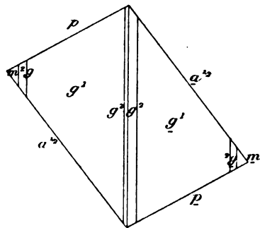
Fig. 22. Macle suivant la loi du Roc Tourné (type 1), silhouette de g^1 (010) 1 .
