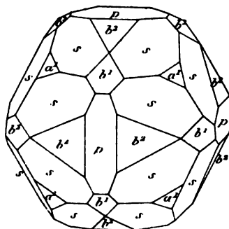
Fig. 17 Pyrite de l'Isère.
