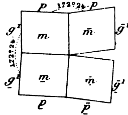
Fig. 4. Projection sur un plan perpendiculaire à l'axe a d'une macle de l'Esterel (figure théorique).
