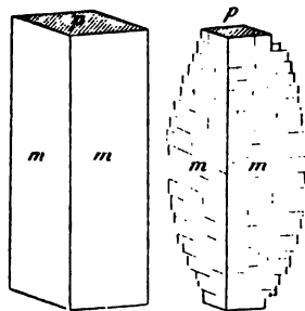
Fig. 5 et 6. Marcasite de Pontpéan (type IV).
