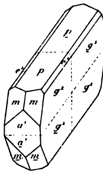
Fig. 4. Stilbite du Mail de Soulan.
