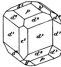
Fig. 2. Proustite de Sainte-Marie-aux-Mines.
