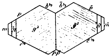
Fig. 13. Macle de Carlsbad avec accollement suivant la face de la zone verticale perpendiculaire à g^1 (010) (Le Freney).
