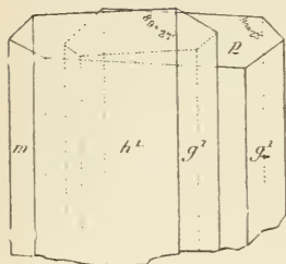
Fig. 3. Macle h^1(100) avec axe de rotation parallèle à l'arête h^1g^1(100)(010) .
