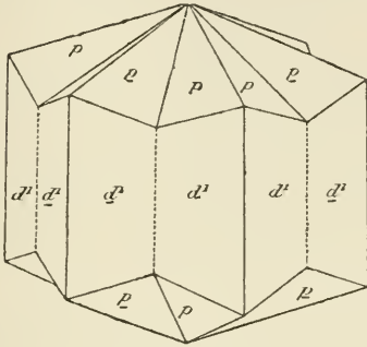
Fig. 5. Phénacite de Framont, maëles avec extrémités symétriques.
