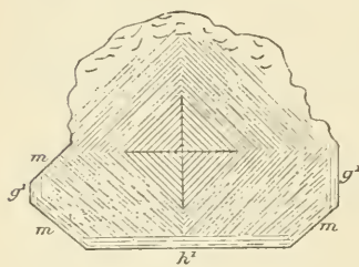
Fig. 4. Lame p (001) de la prehnite de Basse-Indre.
