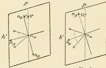
Fig. 1. Plan des axes optiques parallèle à g^1 (010). Angle d'extinction plus petit dans la glaucophane normale (fig. 1) que dans la glaucophane passant à la hornblende (fig. 2).
