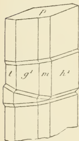
Fig. 4. Macle suivant p(001) et a^{813}(\overline{3}08) .
