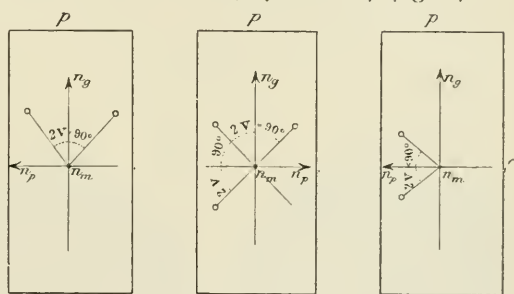
Fig. 1. Enstatite. Fig. 2. Bronzite. Fig. 3. Hypersthène.
