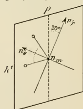
Fig. 1. Plan des axes optiques parallèle à g^4 (010)
