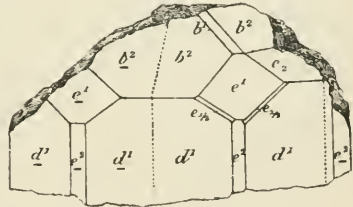
Fig. 8. Phénacite de Framont, maëles sans angles rentrants.
