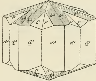
Fig. 5. Phénacite de Framont, maëles avec extrémités symétriques.
