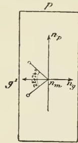
Fig. 2. Plan des axes optiques parallèle à h^1 (100)
