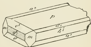
Fig. 7. Epidote de Charmoz.
