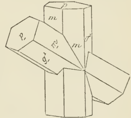
Fig. 6. Macle suivant e^{232}
