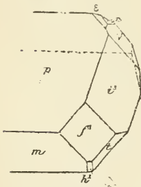
Fig. 2. Axinite de l'Oisans aplatie suivant p (110).
