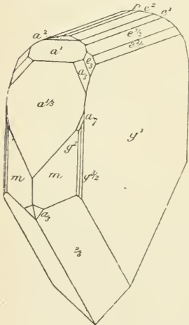
Fig. 5. Calamine de la Vieille Montagne.
