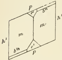
Fig. 5. Epidote de Cabre, projection sur g^1 (010).
