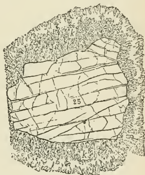
Fig. 31. Coupe mince de grenat (25), présentant la transformation périphérique en spinelle et hypersthène. (Enclave gneissique de la brèche basaltique du Rocher Saint-Michel, au Puy.)
