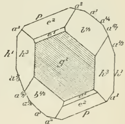
Fig. 11. Epidote du glacier d'Argentièrre, projection sur g^1 (010) .
