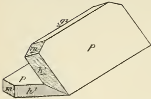
Fig. 12. Bertrandite, macle suivant e^{4/3} (031).
