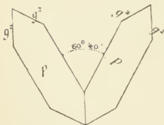
Fig. 7. Bertrandite, macle suivant g^2 (130).
