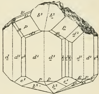
Fig. 7. Phénacite de Framont, maëles à extrémités dissymétriques.
