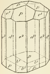
Fig. 13. Tourmaline de Montjeu.
