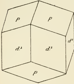
Fig. 1. Phénacite de Framont.
