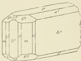
Fig. 6. Idocrase du col de Bousps, allongée suivant l'arête de zone ph^1(001)(100) .
