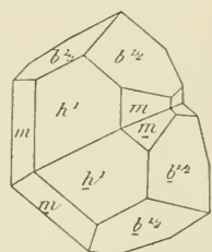
Fig. 6. Augite, macle suivant \bar{l}^1 22 .
