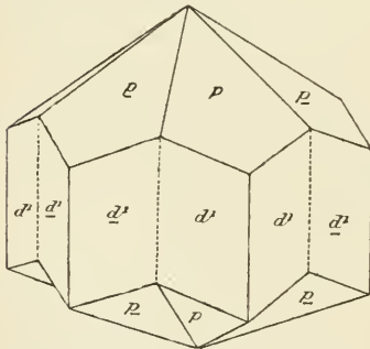
Fig. 4. Macles à extrémités dissymétriques de la phénacite de Framont.
