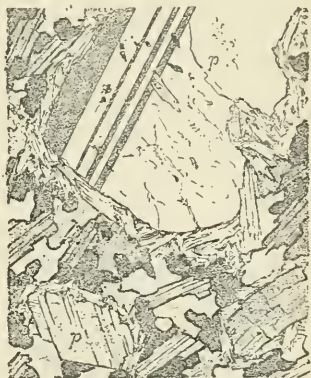
Fig. 8 . Disthène (p) maclé suivant p (001) dans micaschiste de Fay. Il se transforme en damourite à sa périphérie.
