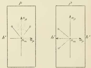
Fig. 1. Anthophyllite. Fig. 2. Gédrite. Plan des axes optiques parallèle à g 1 (010), montrant la position de la bissectrice aigüe .
