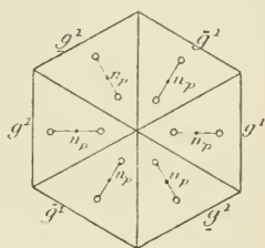
Fig. 2 et 3. Position du plan des axes optiques dans les divers secteurs des cristaux maclés de cordiérite. Face p (001).
