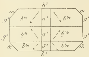
Projection, sur un plan perpendiculaire à l'axe vertical, d'une macle triple, suivant h^1 (100), d'angite des environs du Puy.
