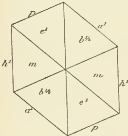
Fig. 6. Epidote de Cabre, projection sur g^1 (010).
