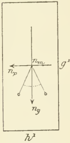
Fig. 1. Plan des axes optiques parallèle à p (001).
