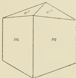
Fig. 16. Pargasite d'Arignac.
