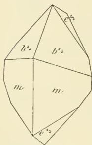
Fig. 8. Fassaïte.
