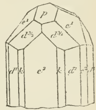
Fig. 19. Tourmaline de Lys
