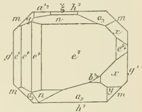
Fig. 7. Projection sur p (001) d'un cristal d'hypersthène du Capucin, remarquable par la dissymétrie du développement des faces du pointement.
