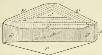
Fig. 14. Tourmaline de Madagascar.
