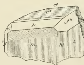
Fig. 30. Axinite de la Rampe des Commères.
