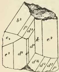
Fig. 9. Fragment d'un cristal de phé- nicite de Framont.
