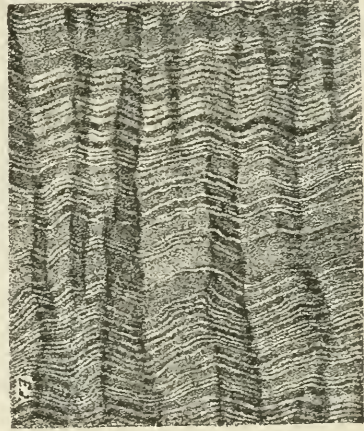
Fig. 1. Lame mince de la métaxite de Moneaup montrant les zones d'accroissement (Lumière polarisée).
