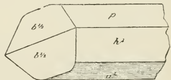
Fig. 12. Epidote du glacier d'Argentièrre.
