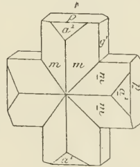
Fig. 5. Macle suivant e^{2/3} (032).
