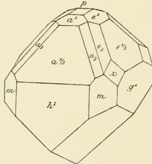
Fig. 6. Calamine de la Vieille Montagne.
