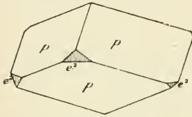
Fig. 3. Phénacite de Framont.
