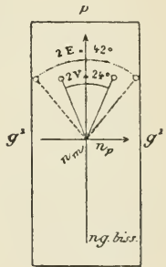
Fig. 3. Plan des axes optiques parallèle à h^1 (100).
