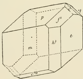
Fig. 21. Axinite de l'Oisans.
