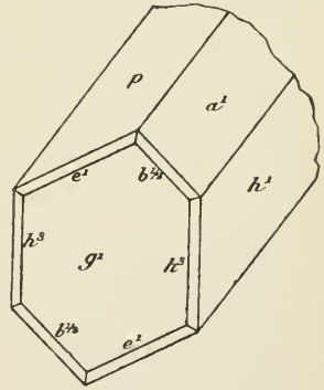
Fig. 14. Epidote du Cornillon.
