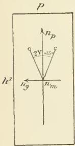
Fig. 1. Plan des axes optiques parallèle à g^1 (010).
