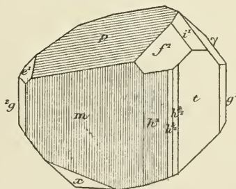
Fig. 30. Axinite de la Rampe des Commères.
