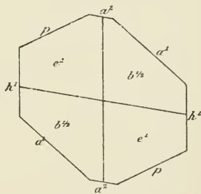
Fig. 3. Épidote d'Illéou, projection sur g^1 (010).
