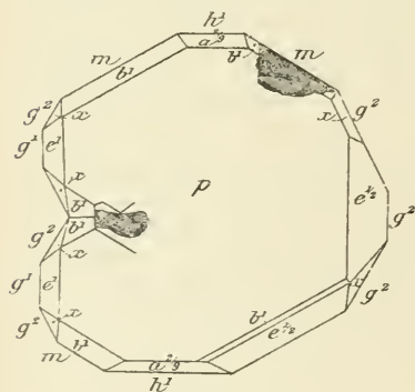
Fig. 10. Pinite d'Isserteaux.
