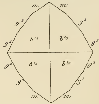
Fig. 1. Projection sur la base d'un cristal d'ilvaïte de Dou-Garoune.
