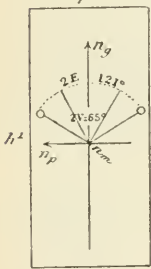
Fig. 1. Plan des axes optiques parallèle à g^1 (010).
