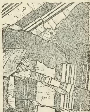
Fig. 10. Lame mince du disthène de Fay montrant les macles suivant p (001). (Lumière polarisée parallèle).
